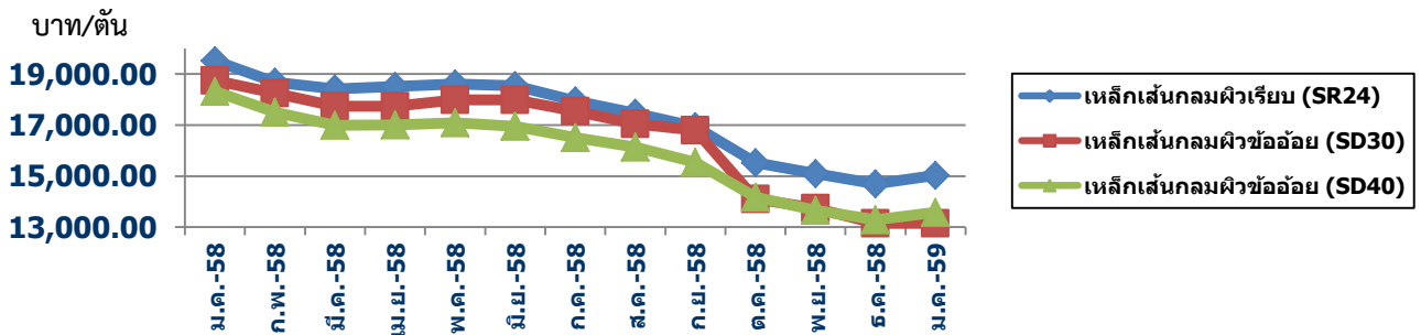
กราฟแสดงแนวโน้มราคาเหล็กเส้นกลมผิวเรียบ SR24 เหล็กเส้นกลมผิวข้ออ้อย SD30 และ SD40
